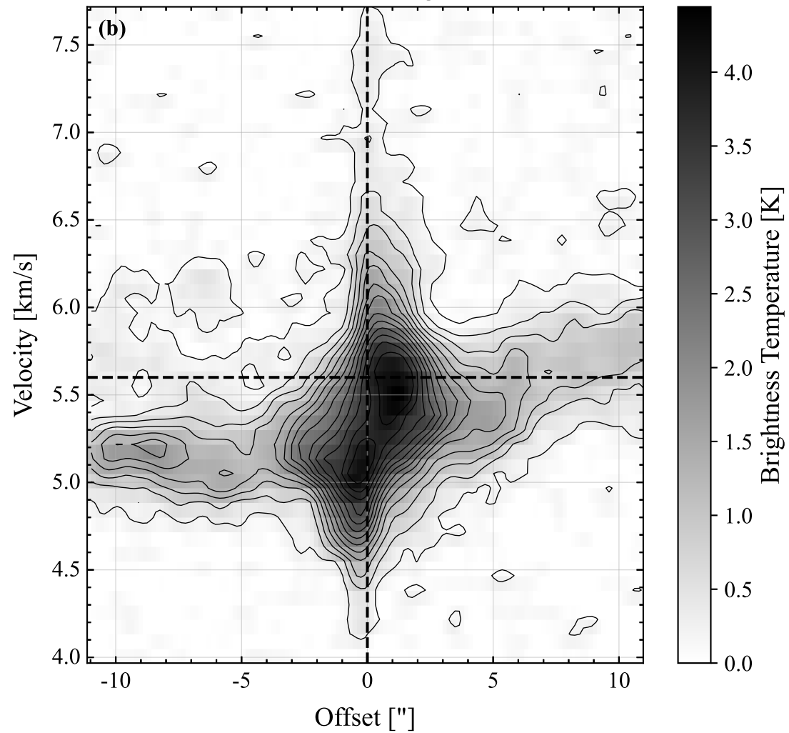
\text{H}_2\text{CO} PV Diagram
